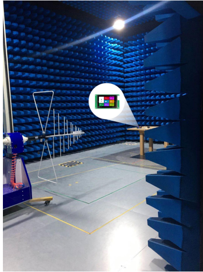
图 5-5 辐射测试图
